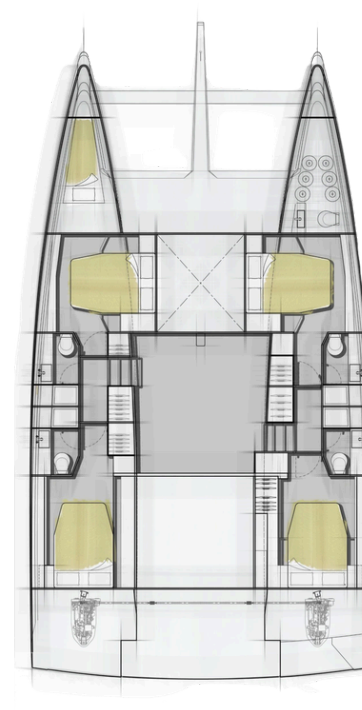
Convés inferior / opção 4 suítes
